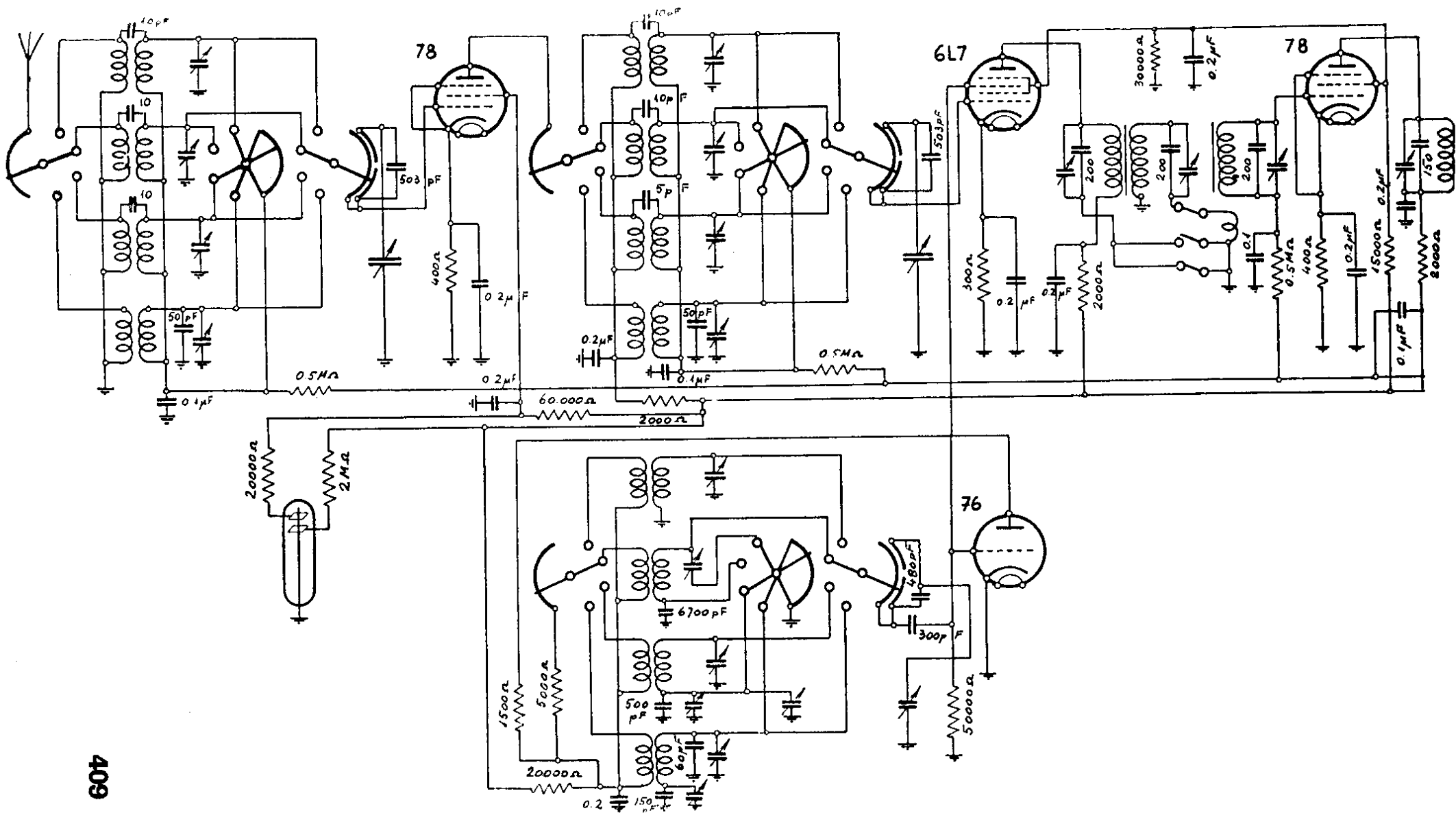
RADIO SAFAR. — Mod. « 844 » e « 940 ». — Parte amplificatrice ad alta e media frequenza (V. nelle pagine seguenti le altre parti). Media frequenza: зНк 094 — Gamme: c. c. (95-19 MHz), c. (55-10 MHz), m. (520-1500 kHz), l. (140-300 kHz).
